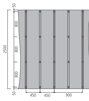
Rozmístění vrtů a podložek na rastru 450 mm pro desky BA12,5 mm šíře 900 mm - desky XL
