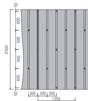
Rozmístění vrtů a podložek na rastru 300 mm pro desky BA12,5 mm šíře 1200 mm - desky XXL
